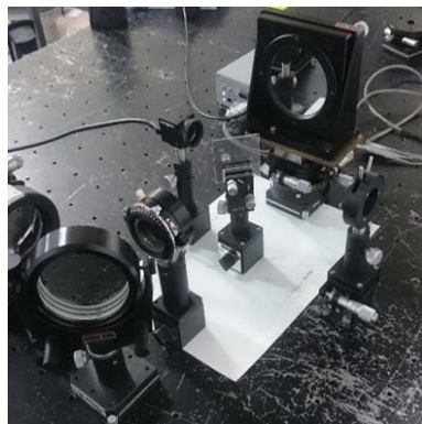
デジタルホログラフィ実験装置
