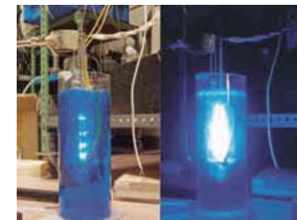
水中における放電プラズマの発生
